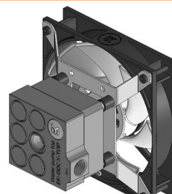
XTOP DDC on vertical FAN
