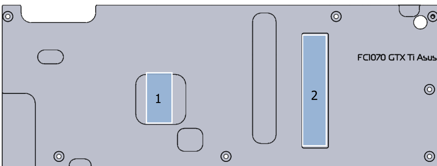
EK-FC 1070 GTX Ti ASUS Backplate
