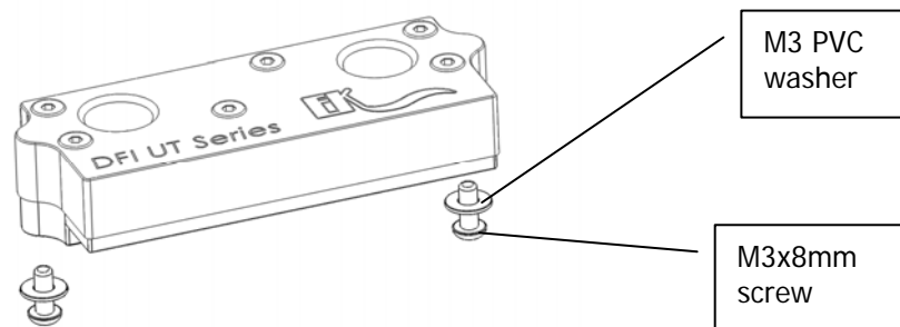
Mosfet DFI UT series
